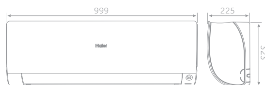
MONTAGEABMESSUNGEN
