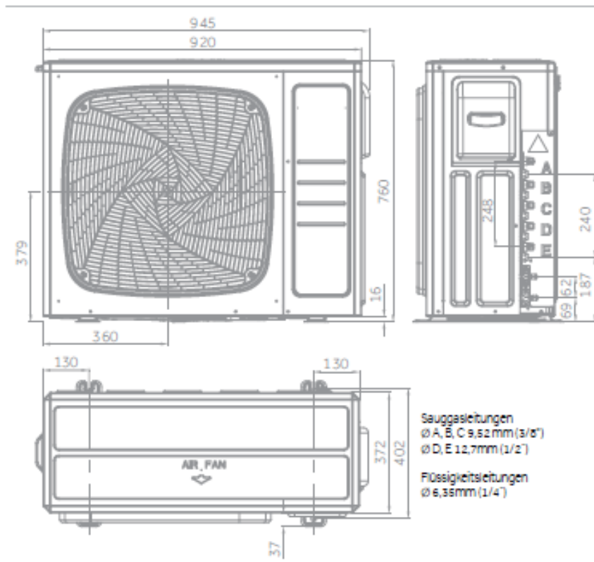
5U90S2SS2FA (5 Kupplungen)
